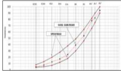
Gambar 4.1 Grafik hasil gradasi agregat gabungan
