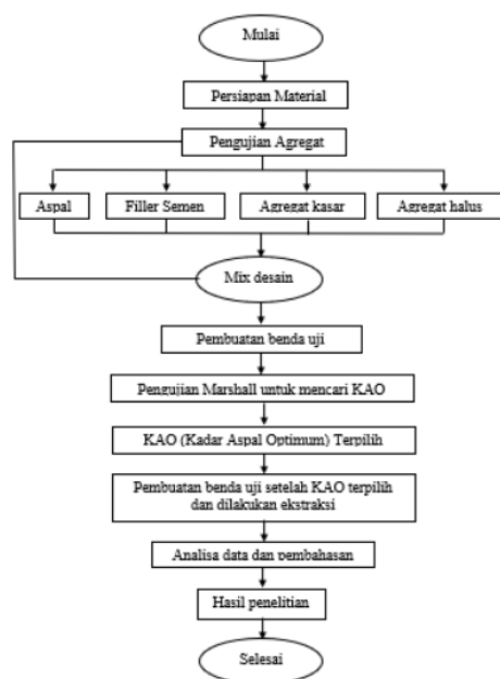
Gambar 3.1 Bagan alir penelitian
