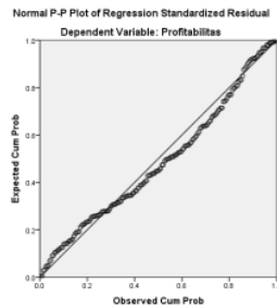
Gambar 1. Uji Normalitas dengan Grafik Normal P-P Plot
