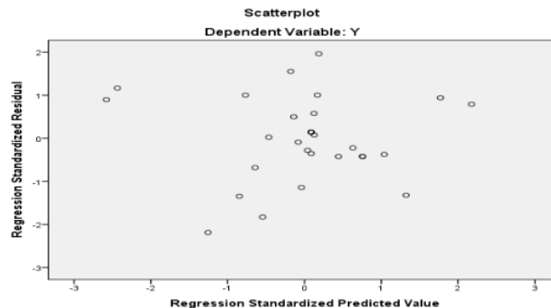
Gambar 2. Uji Heteroskedastisitas
