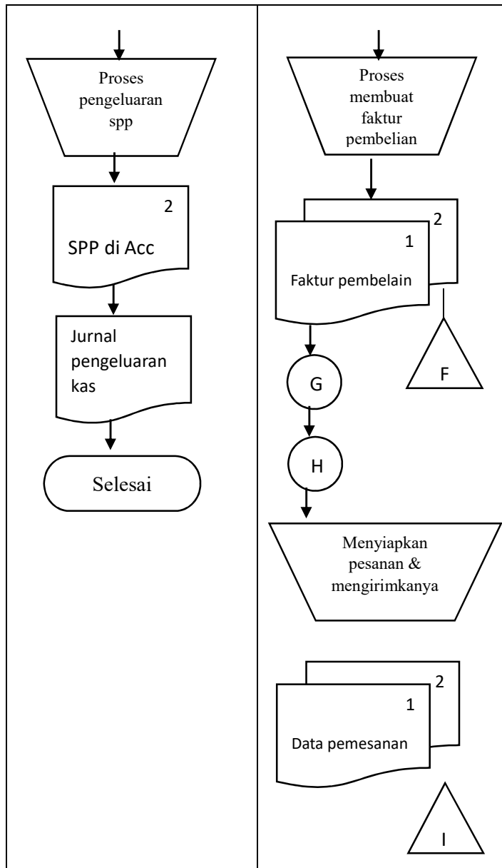
Gambar 3.2 Flowchart Pembelian
