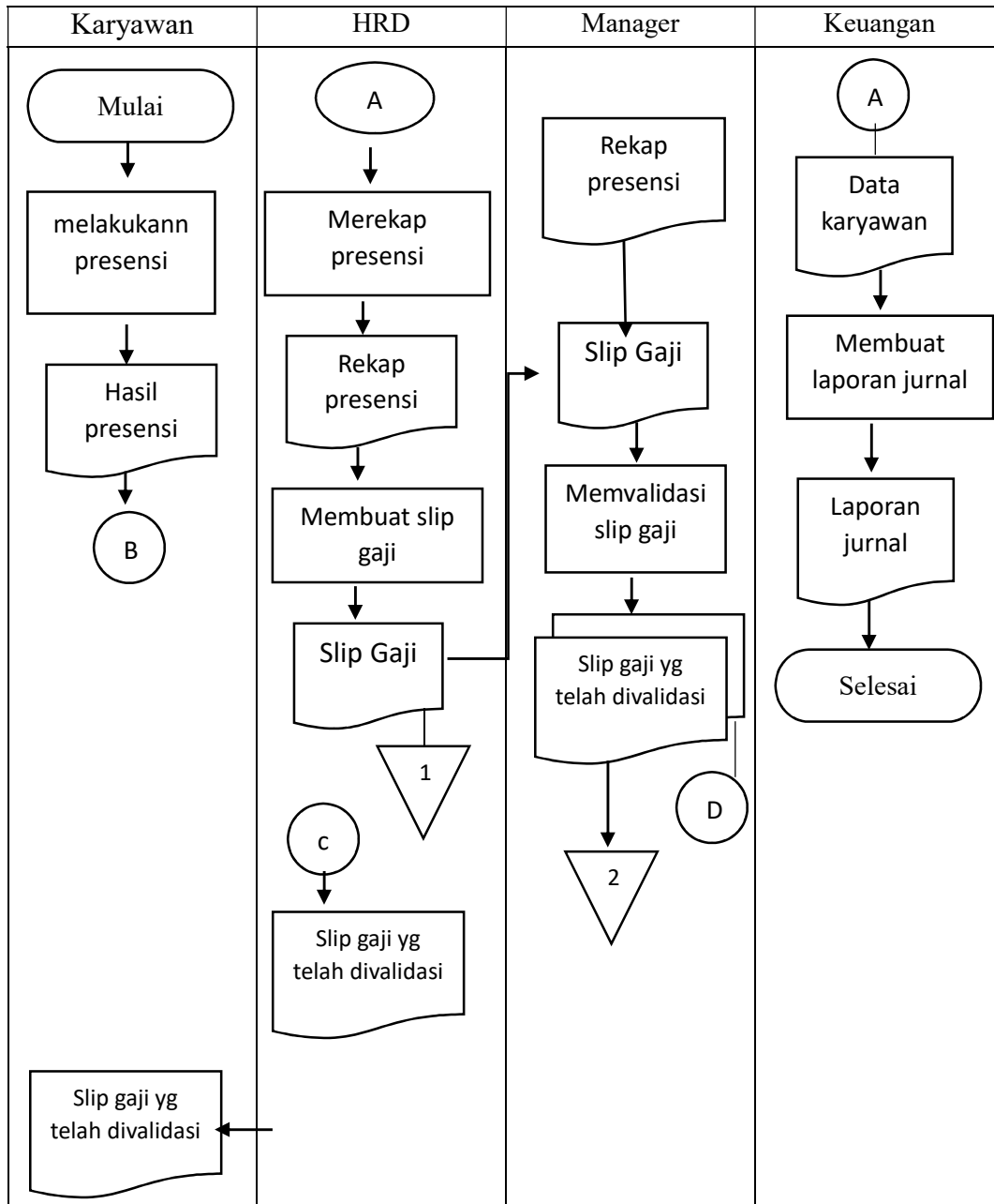
Gambar 3.3 Flowchart Penggajian
